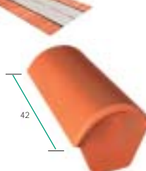
Faitière d'about de 42 (début et fin)
